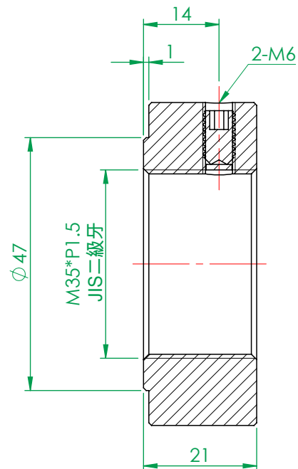
剖面圖 O-O
